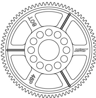
Spur gear 48P 80T 大直齒 230068
