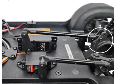
Hauptglockenkurbel
