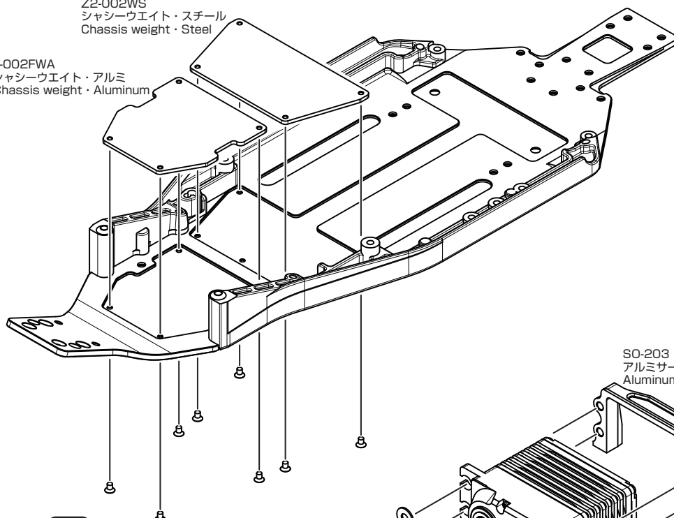
1.5 ZC-F23 M2x3 サラキャップ FHS Screw
