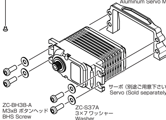
SO-203 アルミサーボマウント Aluminum Servo Mount
